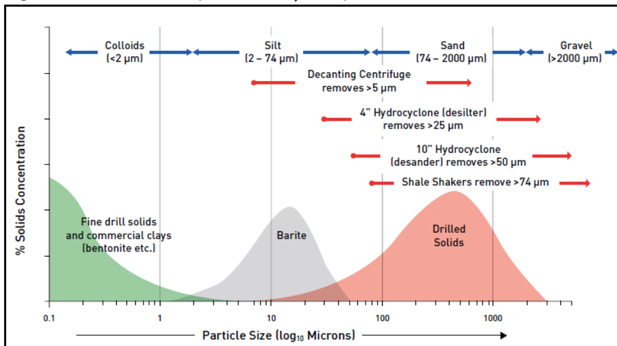
Figura 3.3. Dimensiunile particulelor și echipamentul de înlăturare a solidelor
