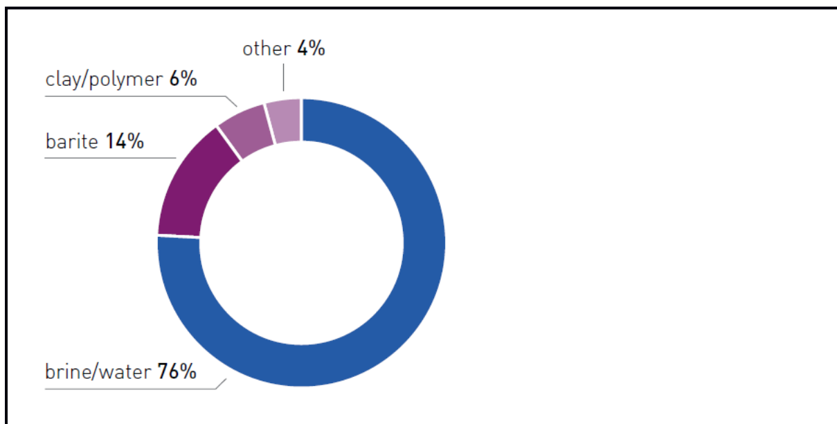
Figura 3.2. Compoziția în procent de greutate a unui WBDGF tipic
