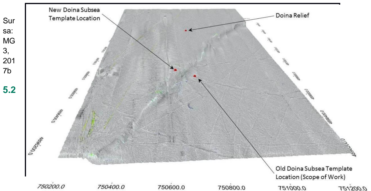
Figura 5.10. Mozaic de imagini scanate cu sonarul lateral în zacământul Doina
